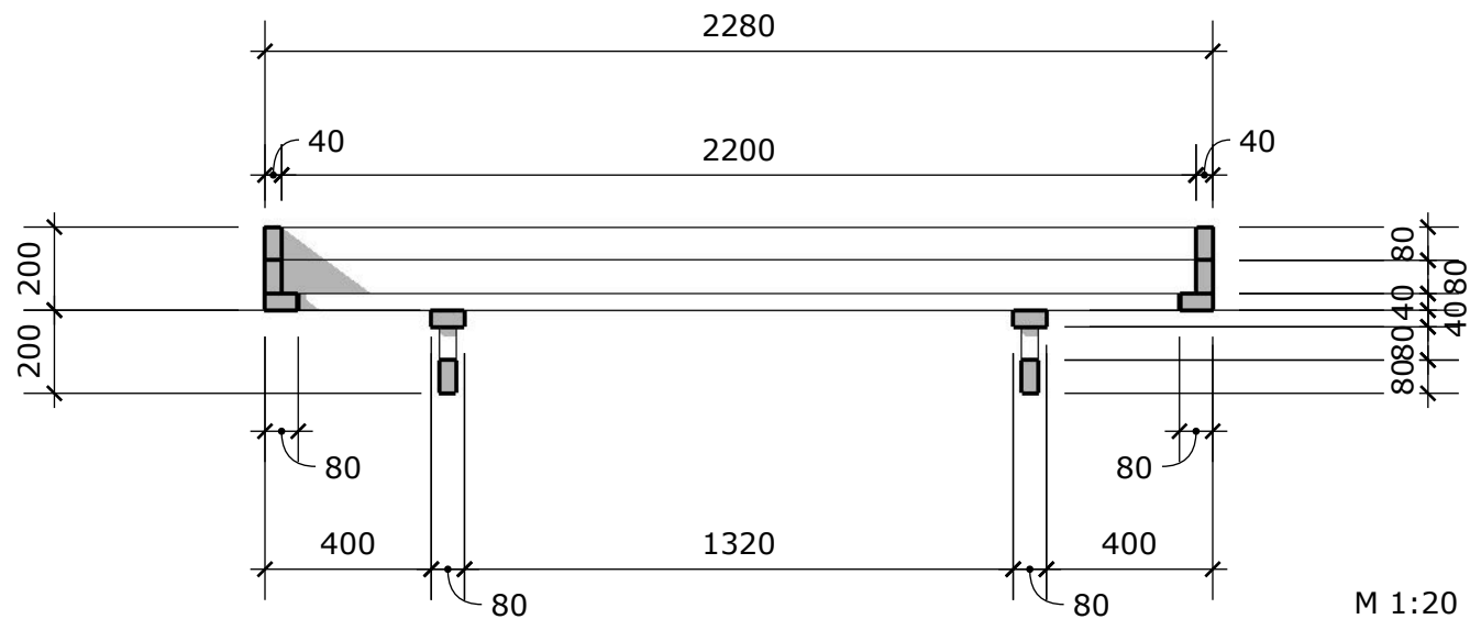
Schnitt A-A (Längsschnitt) / cut A-A (long side)
