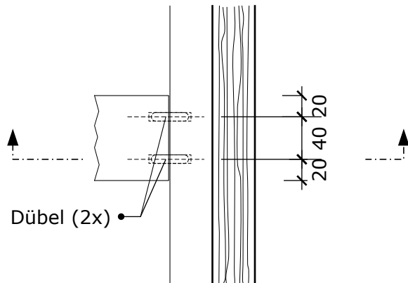
Schnitt horizontal / horizontal cut
