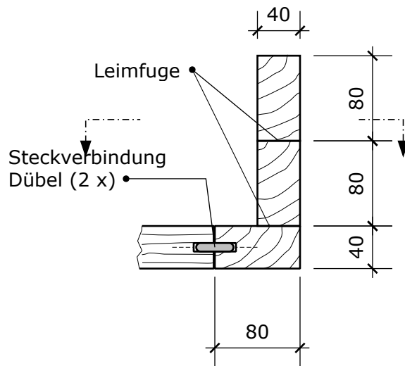
Schnitt vertikal / vertical cut
