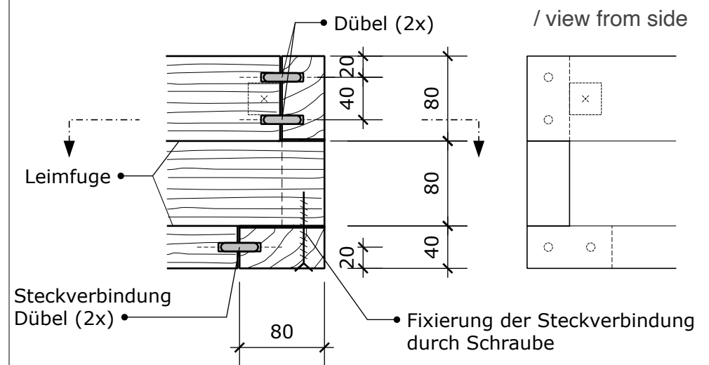
Schnitt vertikal / vertical cut
