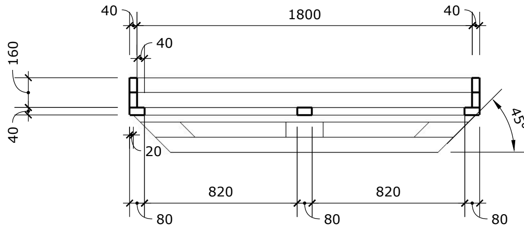
Schnitt B-B (Querschnitt) / cut B-B (short side)
