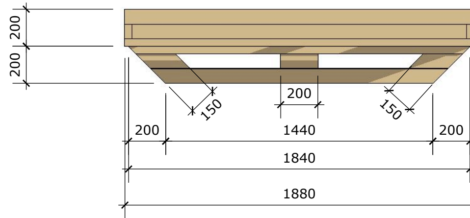
Schnitt B-B (Querschnitt) / cut B-B (short side)
