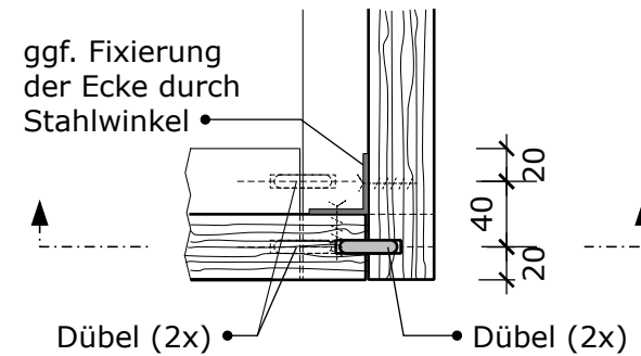
Schnitt horizontal / horizontal cut
