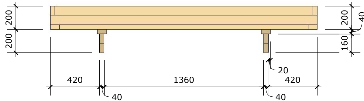
Seitenansicht / view from side
